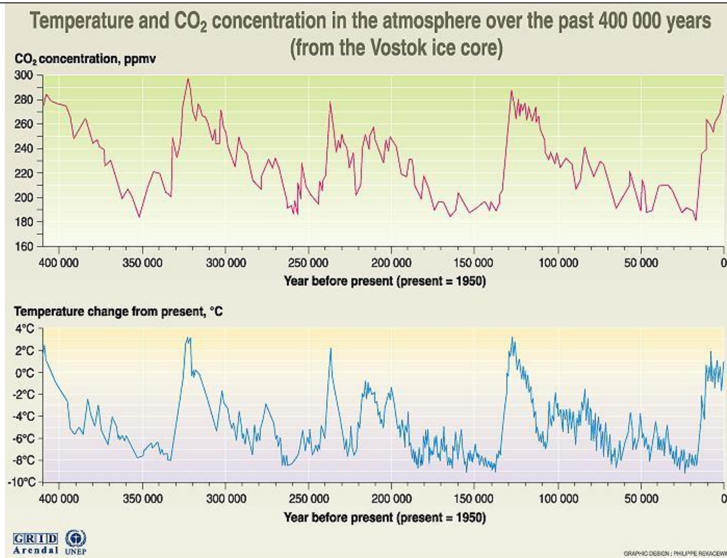
Figur 2: Temperatur og atmosfærens CO 2 -koncentration gennem 400.000
