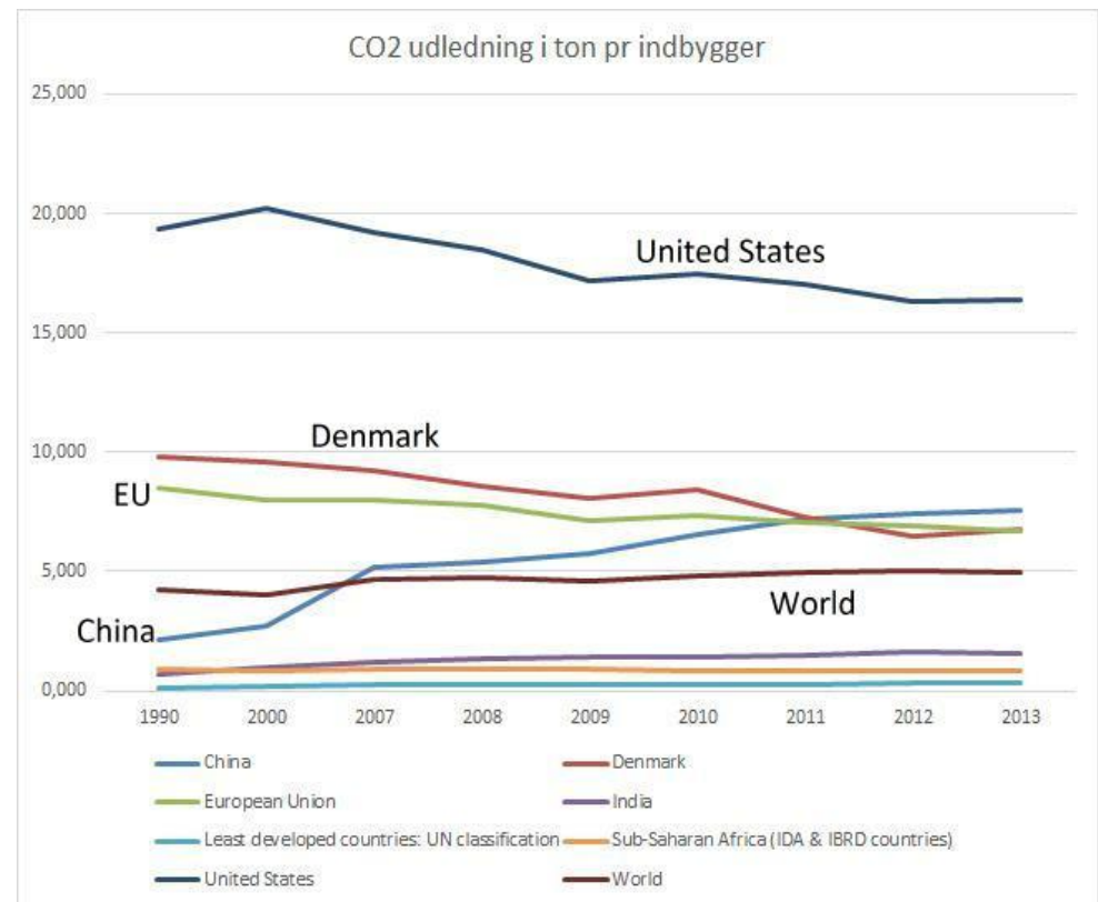
Figur 2 CO2 udledning i ton pr. indbygger
