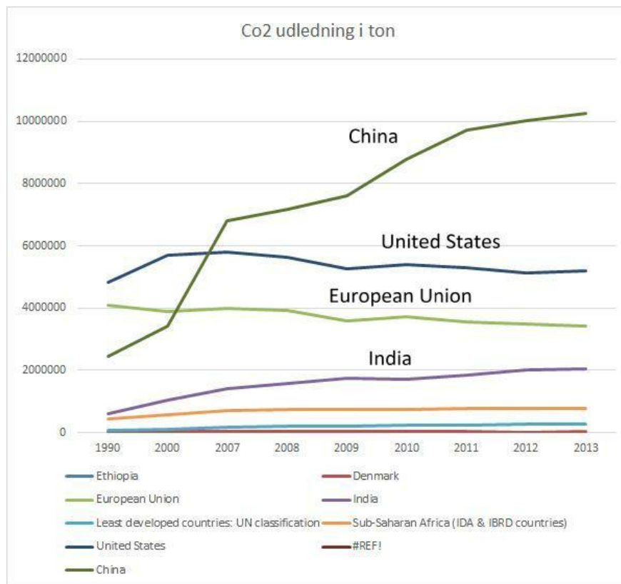
Figur 1 Co2 udledning i ton
